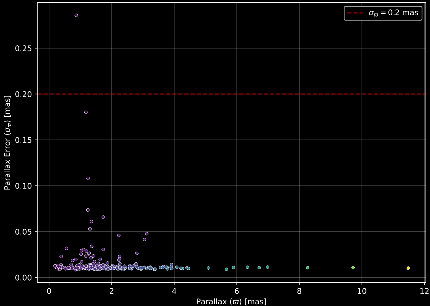
GALAH DR4 Field: [358] Parallax Quality (n= 281)
