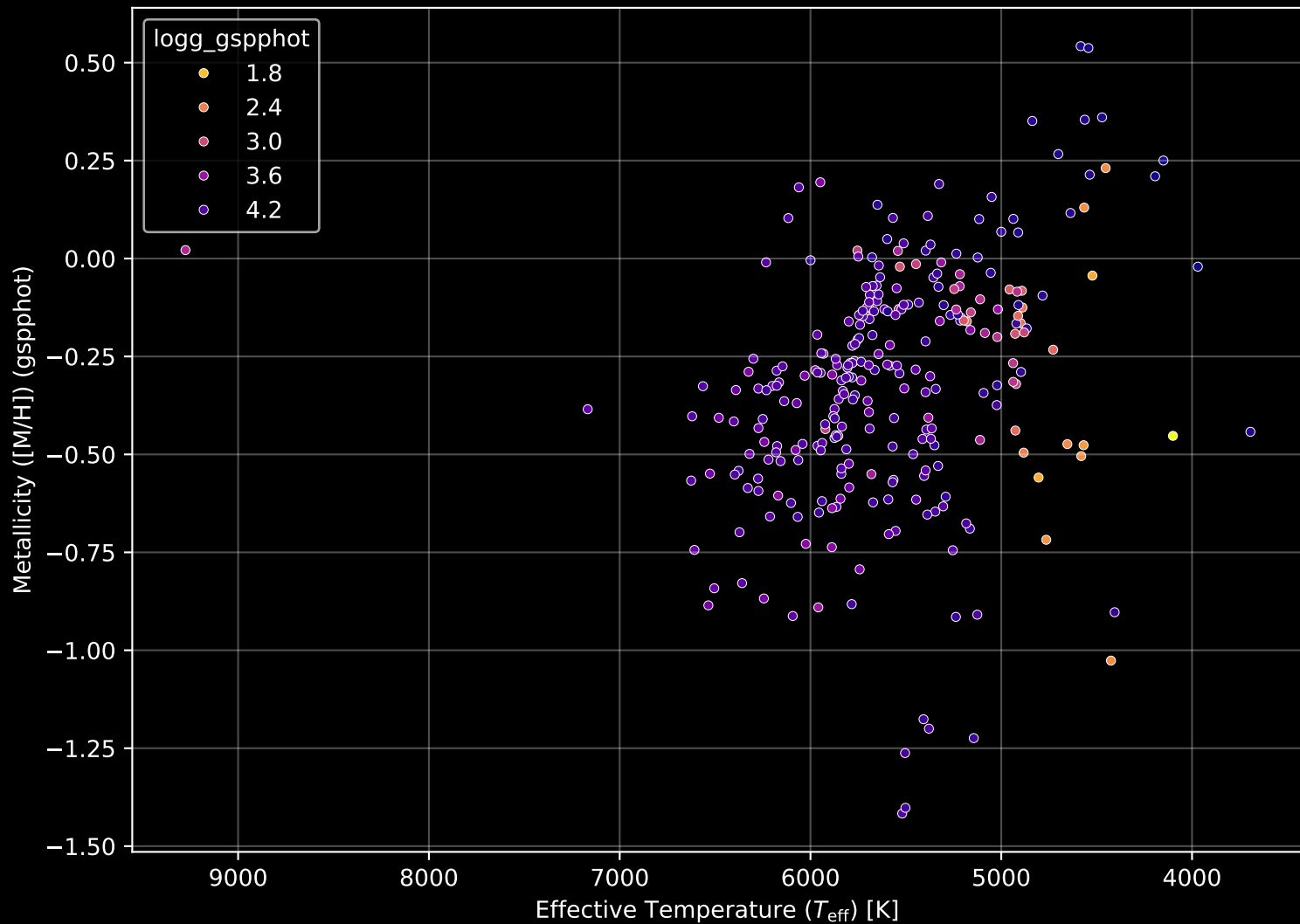
GALAH DR4 Field: [358] Stellar Population Parameters (n= 281)
