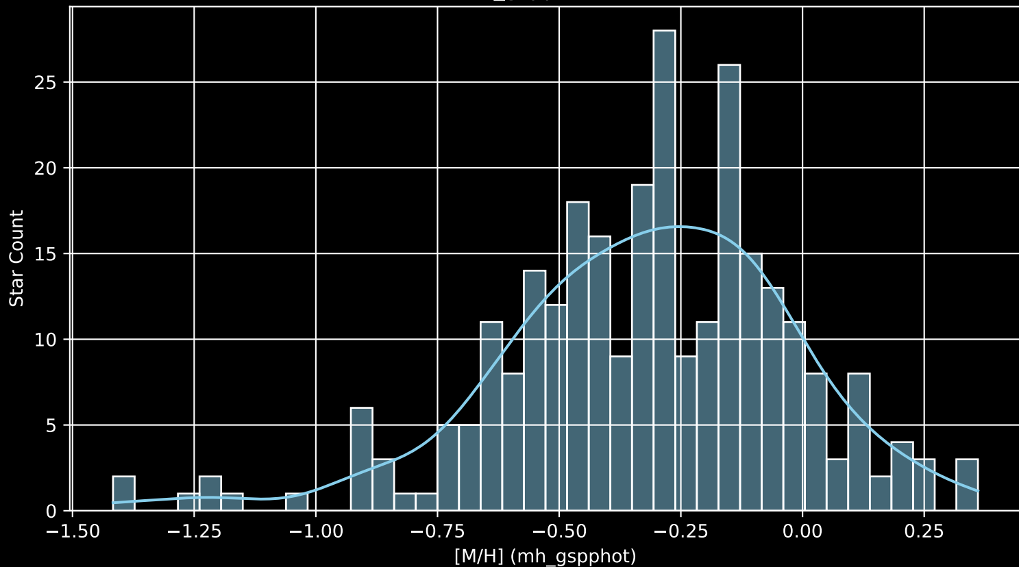
GALAH DR4 Field: [358] [M/H] (mh_gspphot) (n= 279)
