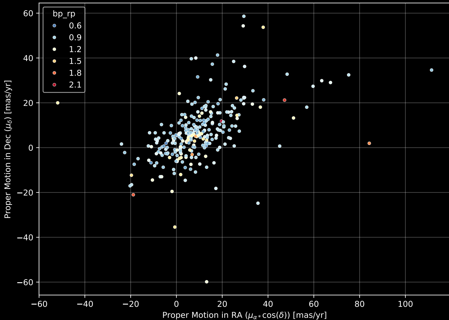
GALAH DR4 Field: [358] Proper Motion Diagram (n= 281)
